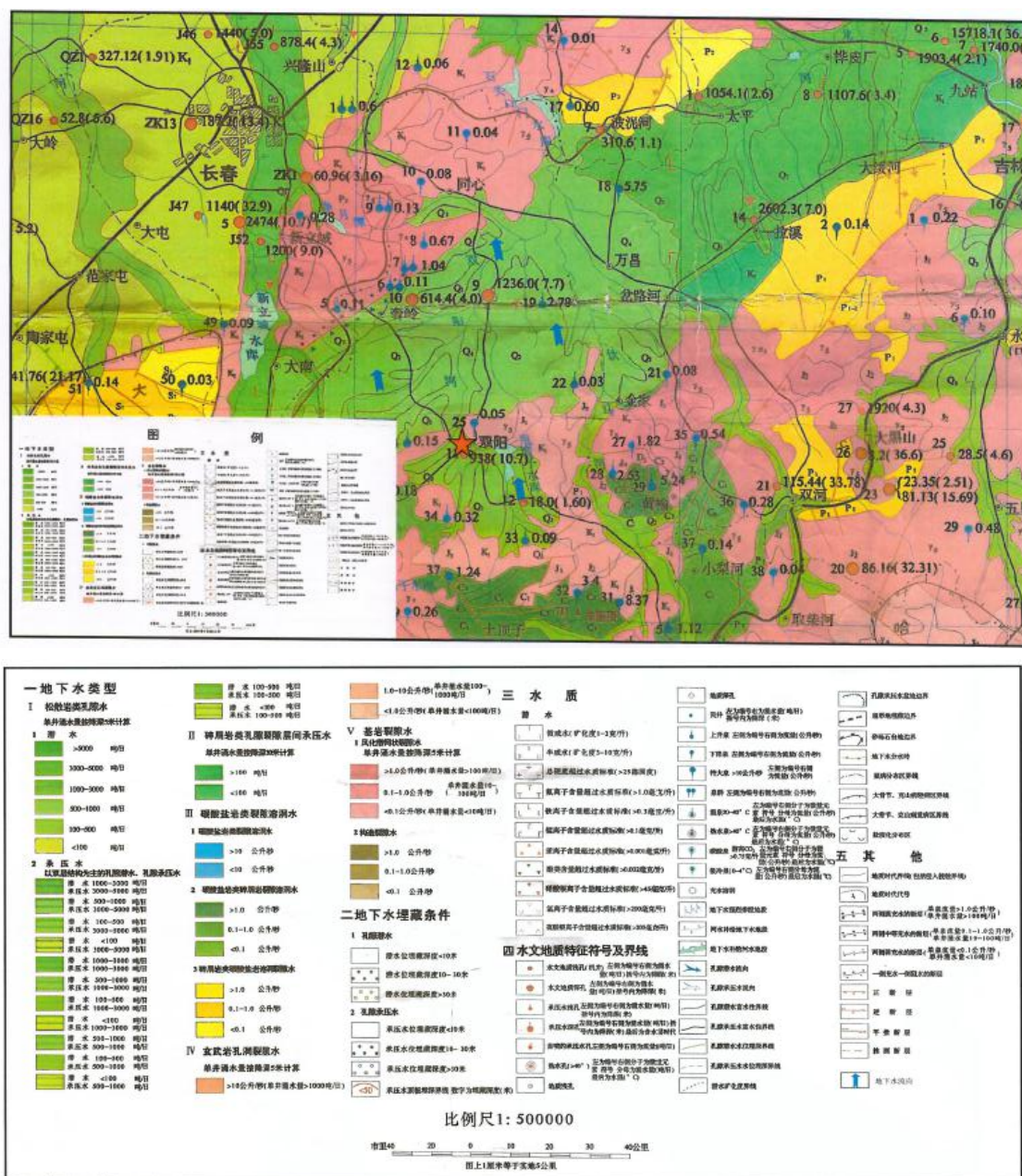
图 2-1 长春市双阳区水文地质图及图例
